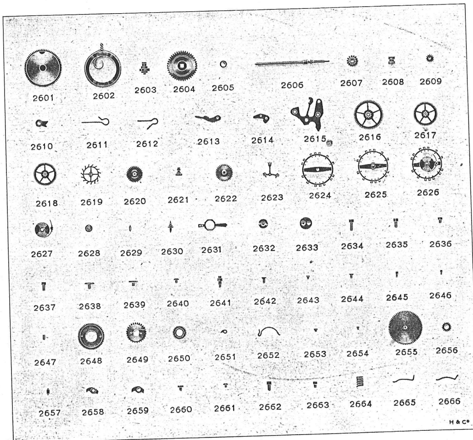
Pièces de rechange des Calibres 161/171 (9¼"")
