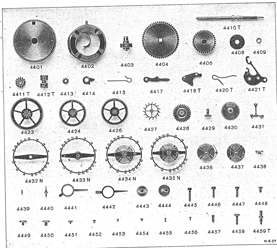
Pièces de rechange du Calibre 433 (16 Size)
