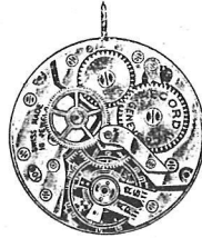
Cal. 106 (10½'''') Seconde au centre
