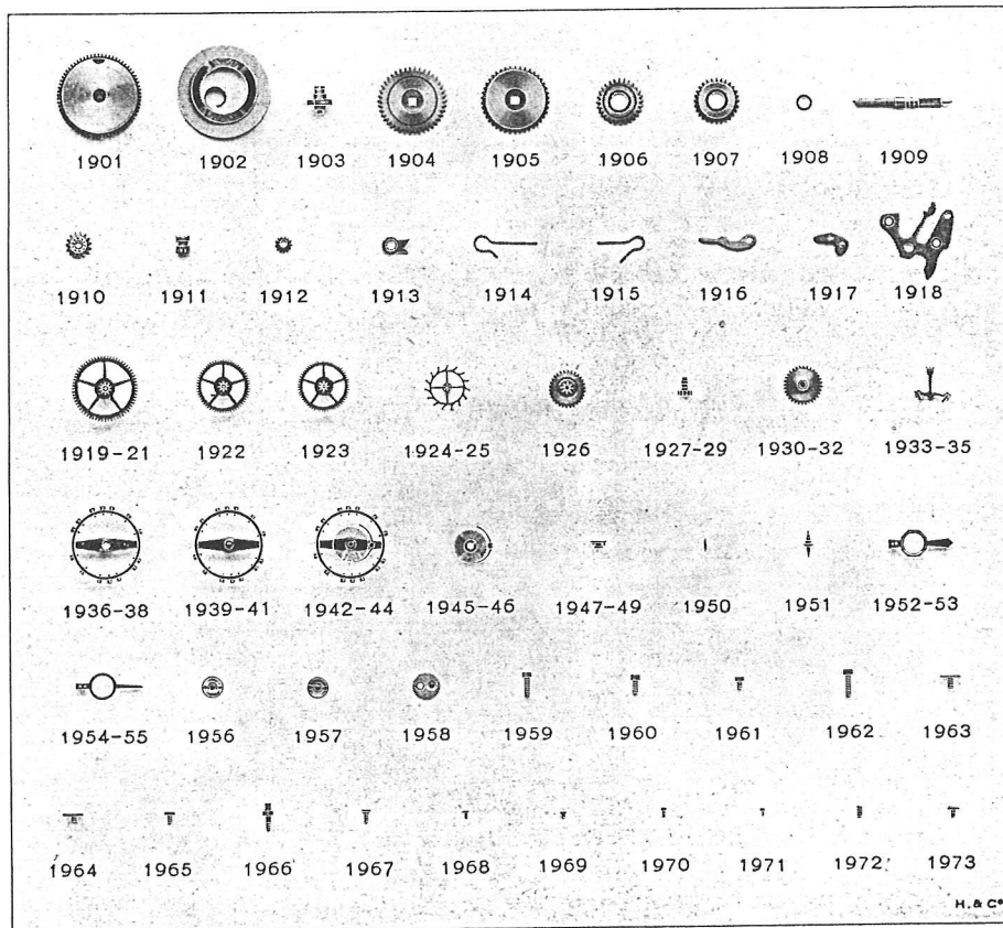
Pièces de rechange des Calibres 160/165 (9¼'''')
