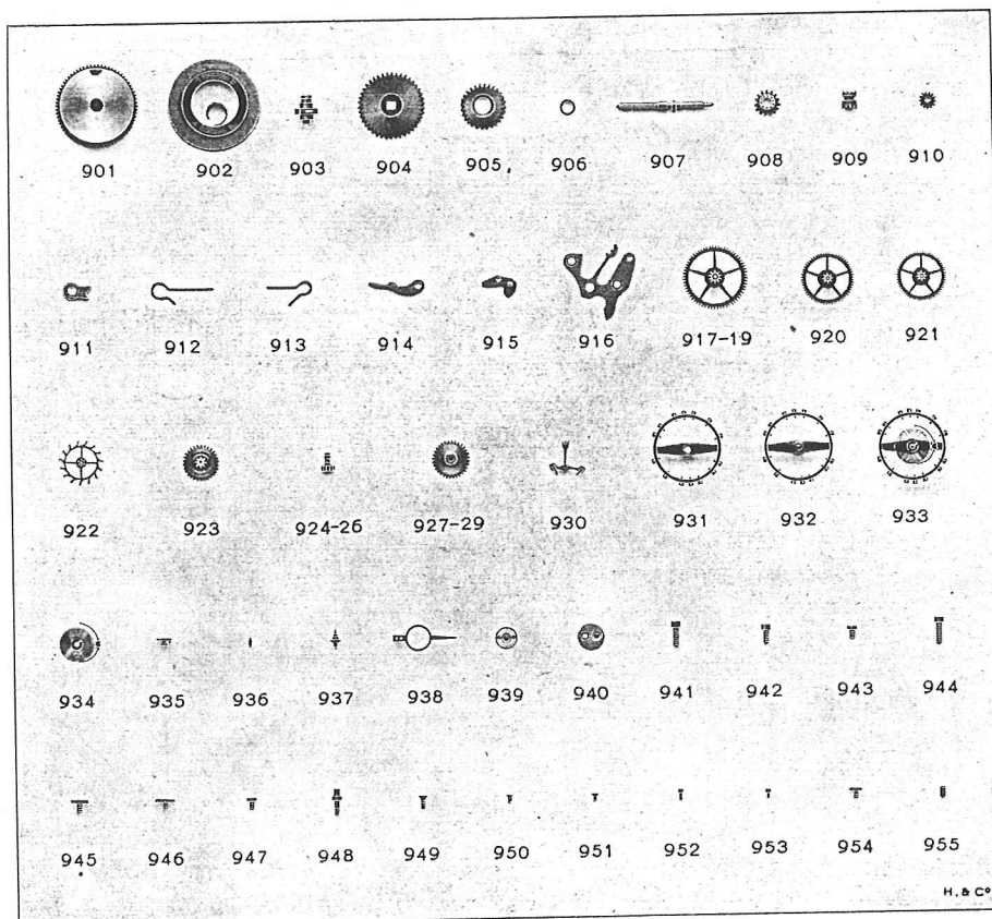
Pièces de rechange du Calibre 170 (9 3/4'''')
