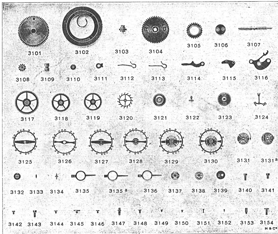
Pièces de rechange du Calibre 022-18 (12½''')
