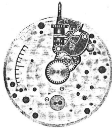
Cal. 022 K (12 1/2''')
