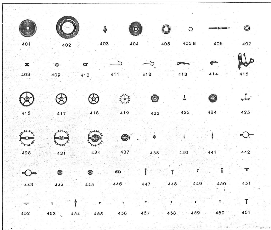
Pièces de rechange des Calibres 50 et 60 (7 \frac{3}{4} ''' )
