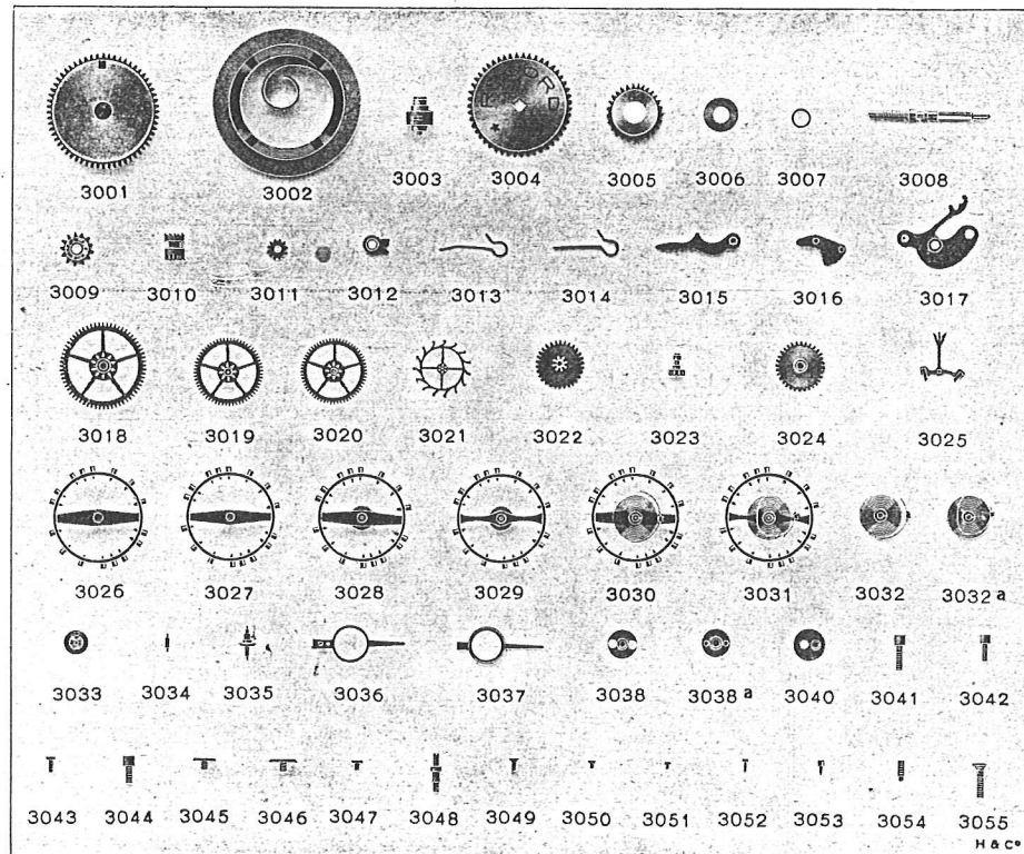
Pièces de rechange du Calibre 022 K (12 1/2''')
