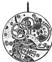
Cal. 170 (9 \frac{3}{4} ''' seconde au centre
