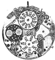
Cal. GCL
