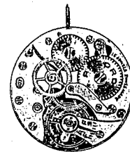
Cal. 107 (10 1/2 mm) Seconde au centre
