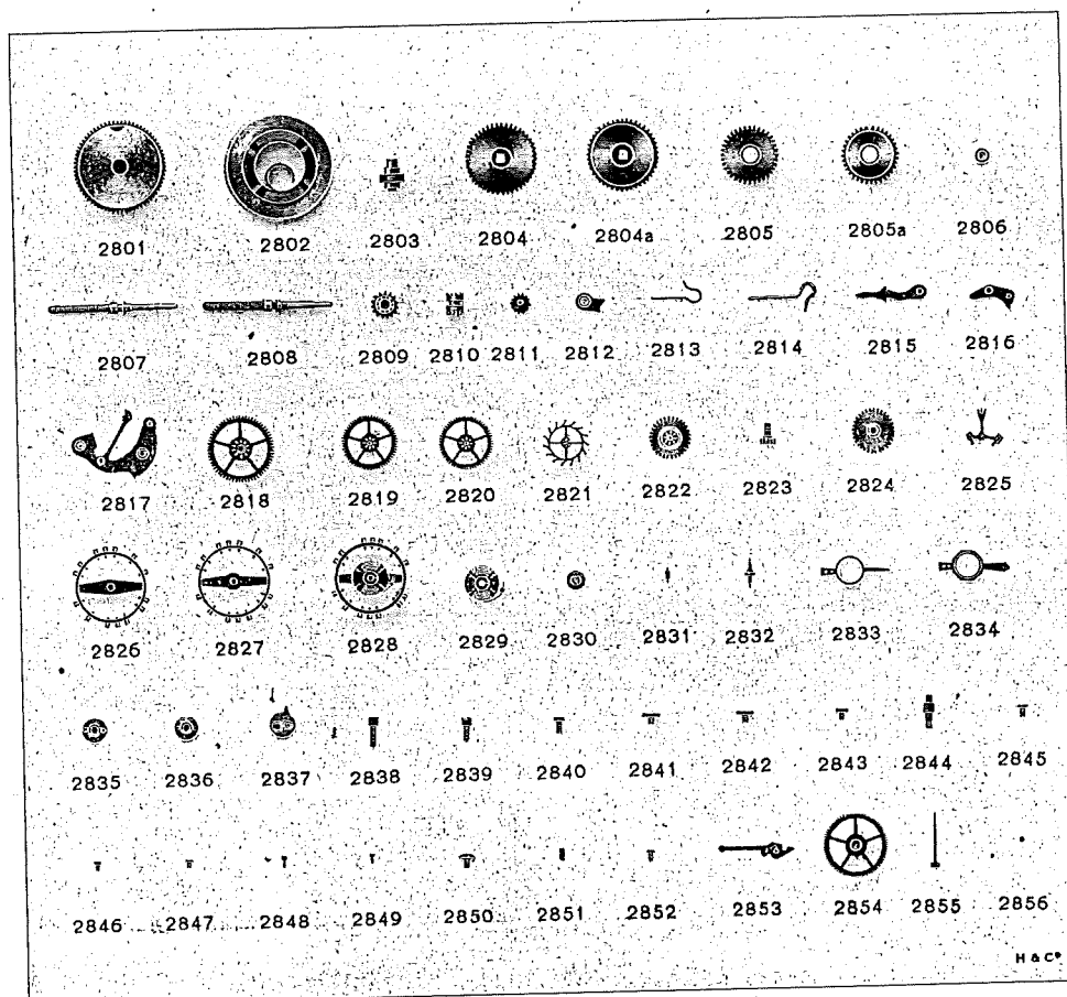
Pièces de rechange des Calibres 106 et 107 (10 1/2 mm)
