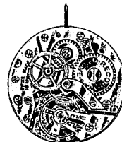
Cal. 160 ( 9\frac{3}{4} "") seconde au centre
