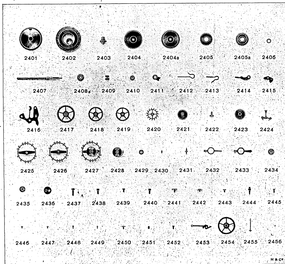
Pièces de rechange des Calibres 160 et 170 ( 9\frac{3}{4} "")
